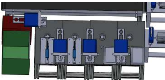
案例 4: 自动在线检测系统 (4 工位在线检测外径, 距离。精度 \pm 0.001\text{mm} )
