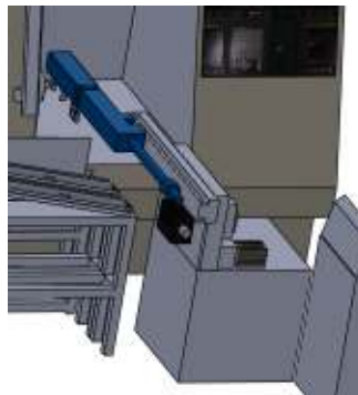
案例 2: 通用数控车床上下料机械手
